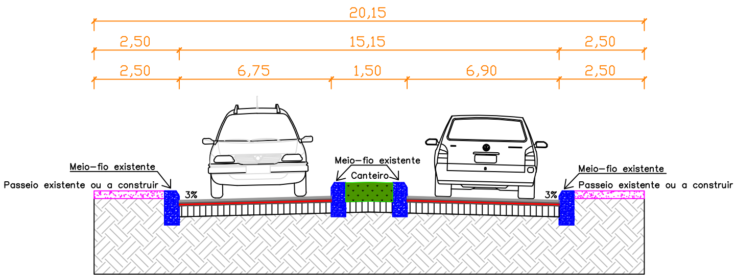
SEÇÃO TIPO DE PAVIMENTAÇÃO NA AVENIDA INDEPENDÊNCIA SEM ESCALA
